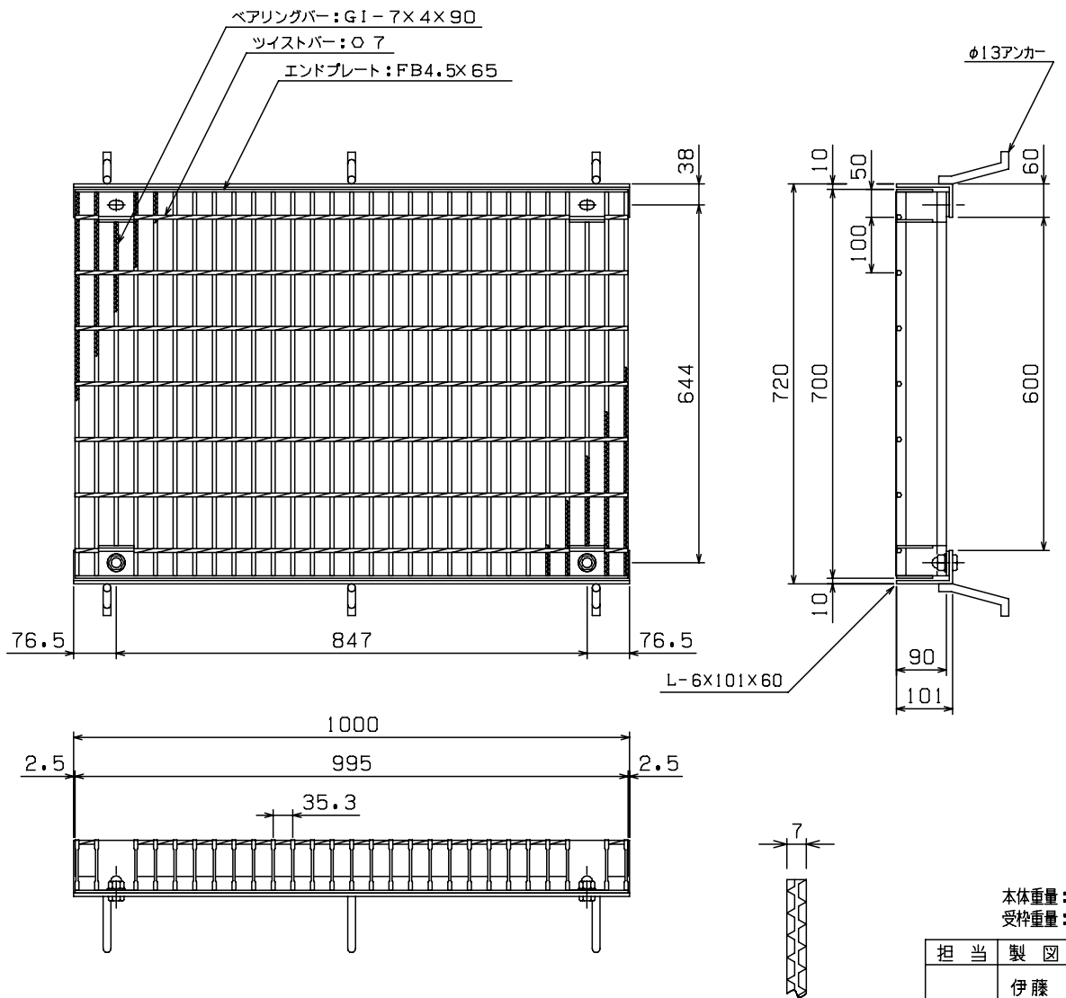
主部材ノンスリップ部詳細
