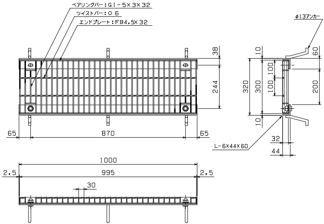
主部材ノンスリップ部詳細
