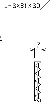
主部材ノンスリップ部詳細
