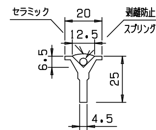
補助部材Yバー部詳細
