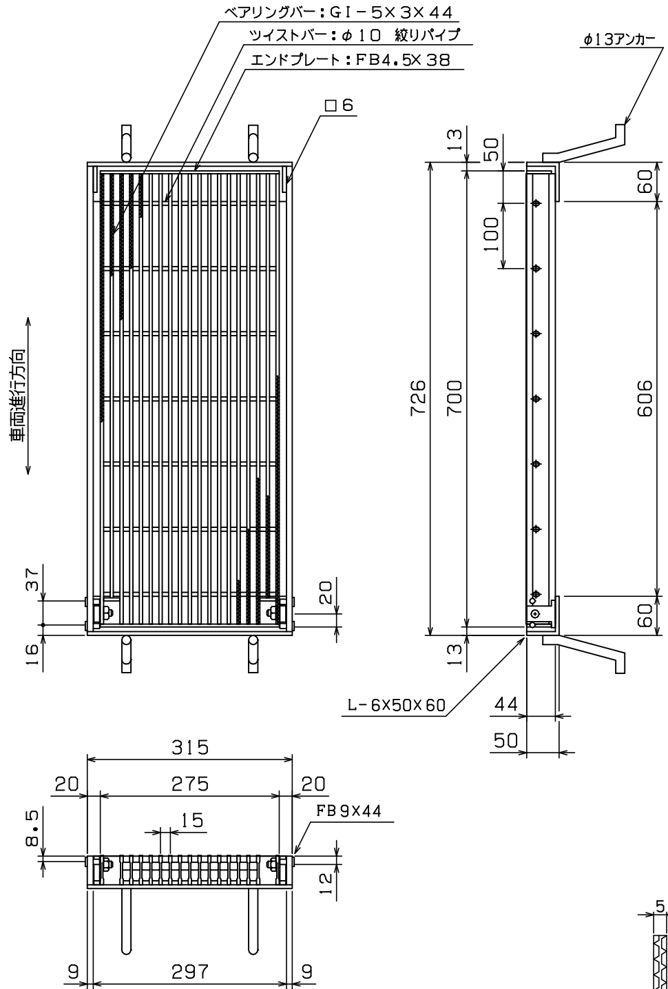
主部材ノンスリップ部詳細
